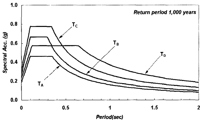
그림 8 재현주기 1,000년 지진에 대한 지반종류별 설계응답스펙트럼
