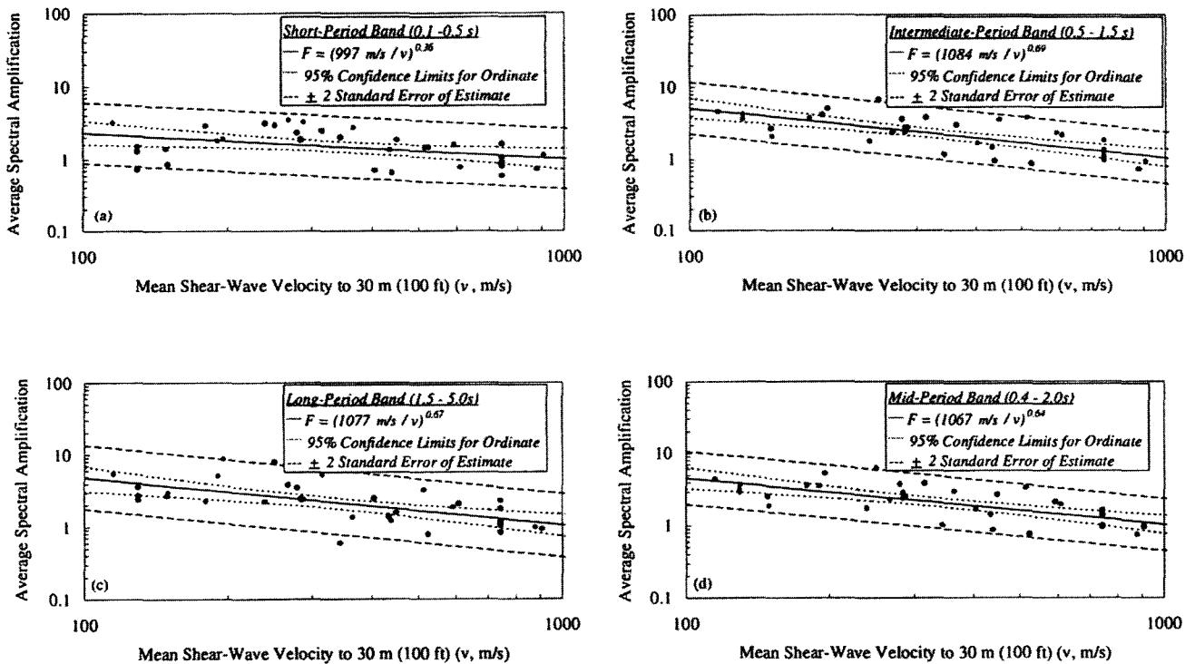
그림 3 다양한 적분구간을 이용한 증폭계수와 V_{s30} 과의 상관관계 (Borcherdt, 1994)
