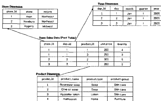
그림 1. 스타스키마 Figure 1. Star Schema
