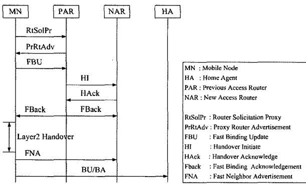
(그림 1) FMIPv6에서 Predictive 모드의 메시지 흐름
