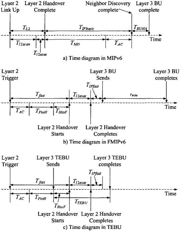
(그림 4) MIPv6, FMIPv6, TEBU 핸드오버 시간도
