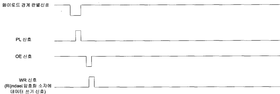
(a) ATM 셀에서 페이로드 데이터 분리 과정 타이밍도
