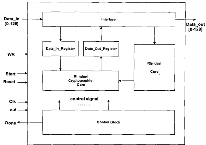
(그림 9) Rijndael 암호화 소자의 구조
