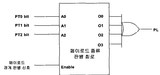
(그림 11) 페이로드 종류 판별 회로
