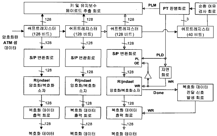
(그림 7) ATM 데이터 보안 장치 수신측 블럭도
