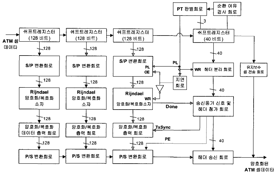
(그림 6) ATM 데이터 보안 장치 송신측 블럭도
