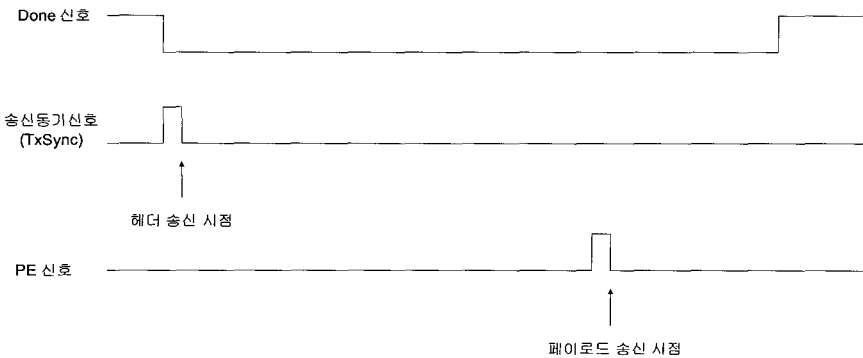
(a) 암호화된 ATM 셀 전송 타이밍도
