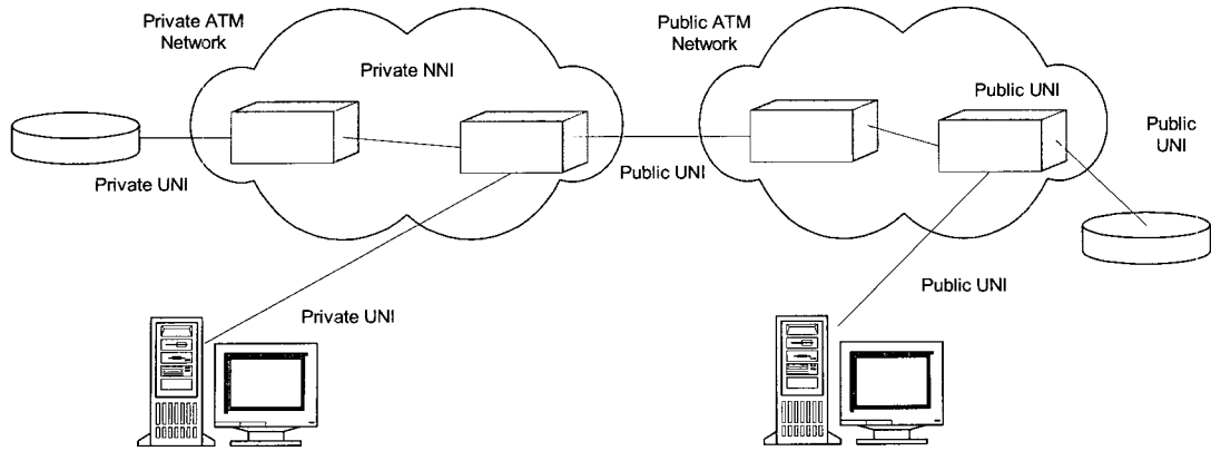
(그림 5) ATM 망의 구조
