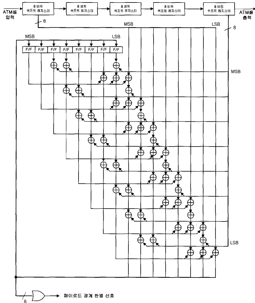
(그림 10) 순환 여유 검사 회로
