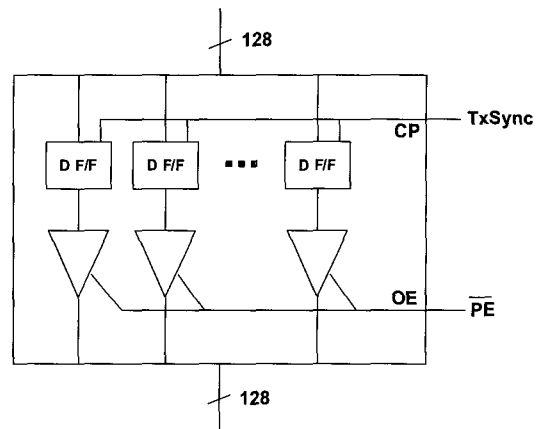
(그림 13) 암호화 데이터 출력 회로
