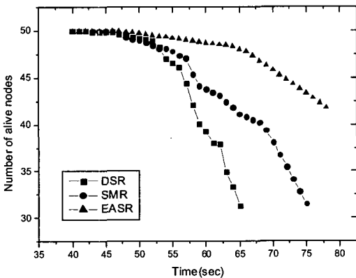
그림 5. 시간에 따른 동작 가능한 노드의 개수
