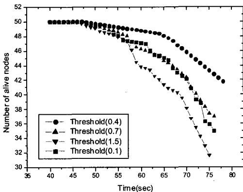
그림 6. Overheard 지수의 임계치 변화에 따른 EASR의 동작 가능한 노드의 개수
