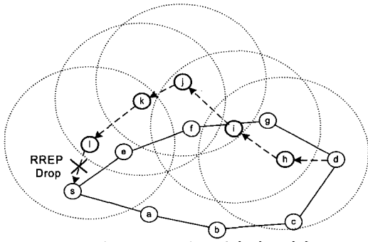
그림 3. EASR의 overhearing을 고려한 경로 선정
