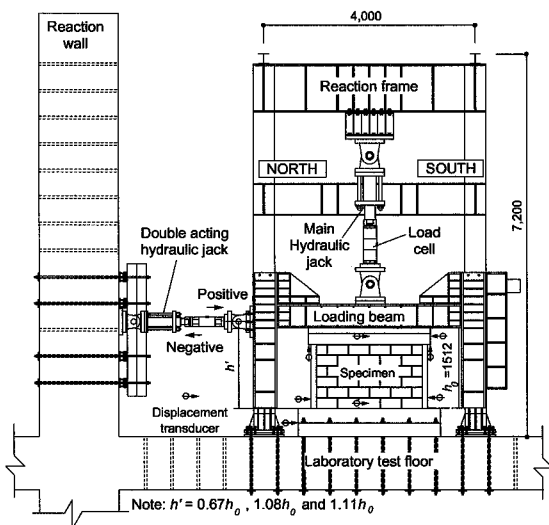
<Fig. 5> Test setup
