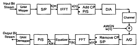
그림 1. 기저대역 OFDM 시스템 모델
