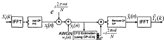
그림 3. AWGN 채널에서의 제안된 CP-ICA를 이용한 주파수 옵셋 추정기
