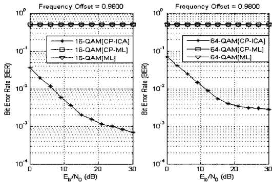
그림 13. ICI가 제거된 BER 곡선, \varepsilon = 0.98
