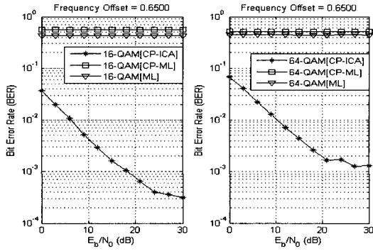
그림 12. ICI가 제거된 BER 곡선, \varepsilon = 0.65
