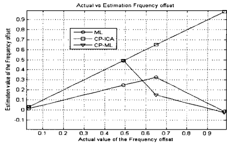
그림 14. 주파수 오프셋 추정기에 따른 주파수 오프셋 추정치, \varepsilon = \{0.032, 0.49, 0.65, 0.98\}
