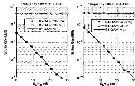
그림 10. ICI가 제거된 BER 곡선, \epsilon = 0.032
