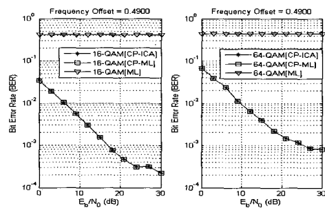
그림 11. ICI가 제거된 BER 곡선, \epsilon = 0.49
