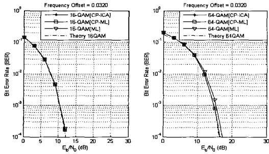
그림 5. ICI가 제거된 BER 곡선, \epsilon = 0.0320
