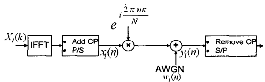
그림 2. 기저대역 주파수 오프셋 모델
