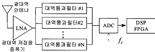
그림 2. 대역통과와 샘플링을 사용하여 N개 신호의 하향변환을 위한 수신기 구조
