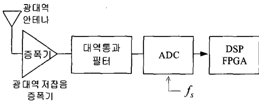
그림 1. 신호 하나의 복조를 위한 SDR 시스템의 수신기모델
