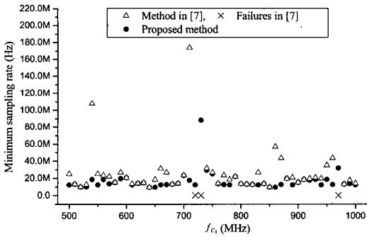
그림 8. 나이퀴스트 율 아래에서 전체 샘플링 주파수 영역의 합을 비교
