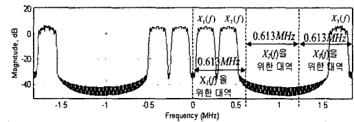
그림 6. f_s = 3.678 \text{ MHz} 에 의하여 샘플링한 스펙트럼
