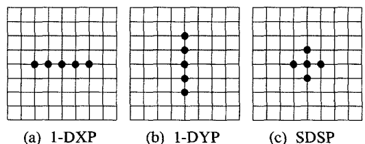
그림 7. 제안하는 알고리즘에서 사용되는 탐색패턴
