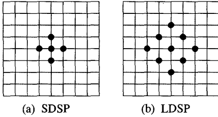
그림 3. 다이아몬드 탐색 패턴
