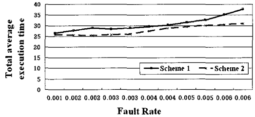
그림 7. Fault rate 변화에 따른 평균 수행시간 비교
