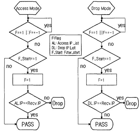
(그림 4) access/drop mode 패킷처리
