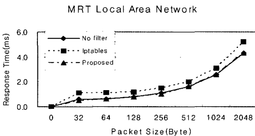
(그림 9) LAN의 최소 응답시간
