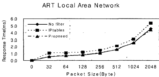
(그림 10) LAN의 평균 응답시간
