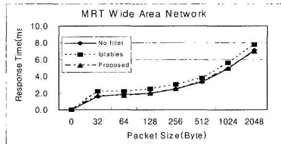
(그림 7) WAN의 최소 응답시간
