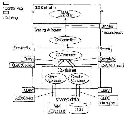
그림 4. 그레이팅배치기 모듈의 설계 Fig. 4. Components of Grating Allocator Module
