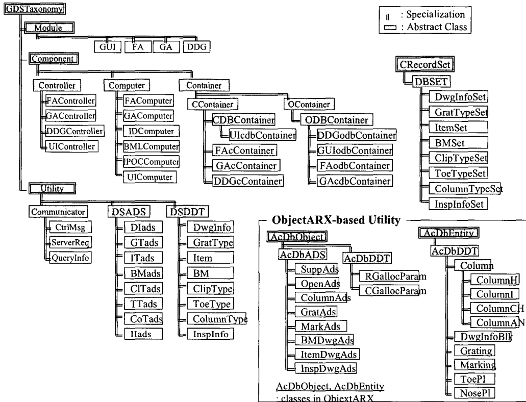
그림 5. 클래스 계층도 Fig. 5. Class Hierarchy
