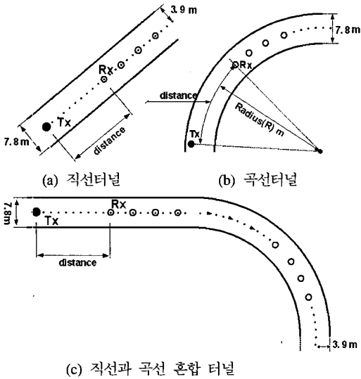
그림 4. 터널의 평면구조 및 송수신기 위치
