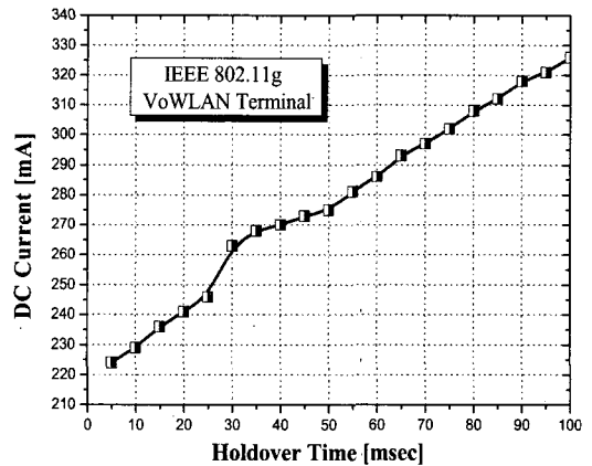
그림 5. VoWLAN 단말기의 Holdover time에 따른 전류 레벨
