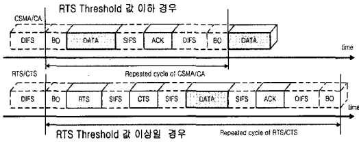
그림 1. RTS/CTS 동작 상태
