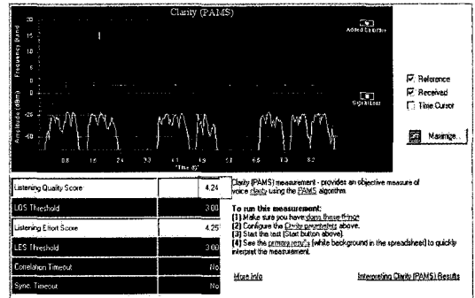
그림 13. 동시 통화 8대에게 가변 Hold over time을 구현한 VQT 측정값
