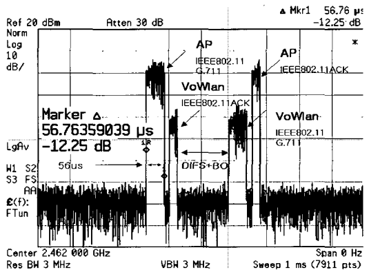
그림 8. PSA로 측정된 AP와 VoWLAN 단말기의 전송 간격 측정
