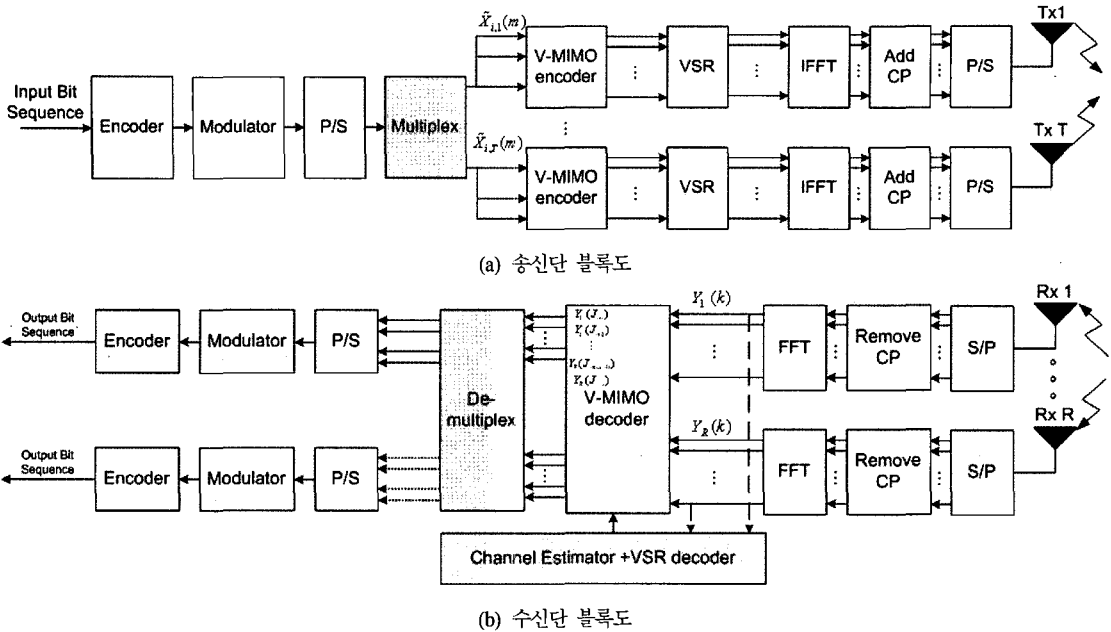
그림 4. MIMO 환경에서의 가상 다중 안테나 기법 블록도 Fig. 4. The block diagram of subcarrier-based virtual multiple antenna system at MIMO
