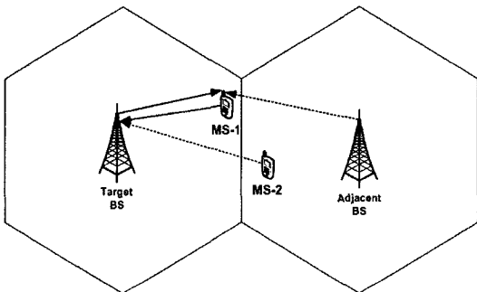
그림 7. 셀룰러 환경에서 인접 셀간의 간섭 Fig. 7. Inter-cell interference at cellular system
