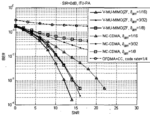
그림 8. 가상 다중 안테나 기법을 이용한 상향링크 SDMA 기법 Fig. 8. The simulation result of uplink SDMA method using subcarrier-based virtual multiple antenna
