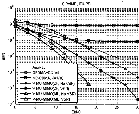
그림 10. 가상 다중 안테나 기법을 이용한 하향링크 ICI 제거 기법 Fig. 10. The simulation result of downlink ICI cancellation method using subcarrier-based virtual multiple antenna
