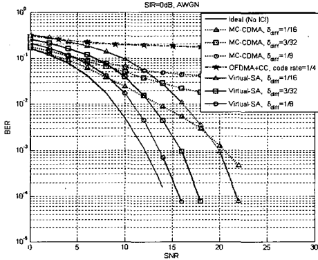
그림 9. 가상 스마트 안테나 기법을 이용한 하향링크 ICI 제거 기법 Fig. 9. The simulation result of downlink ICI cancellation method using virtual smart antenna
