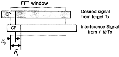
그림 1. 두개의 인접 기지국에서 동시에 수신된 신호 Fig. 1. The received signal form target and interference BS at cell boundary
