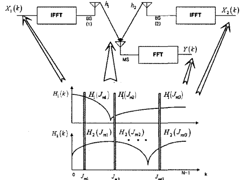
그림 2. 부반송파 기반 가상 다중 안테나 시스템 개념도 Fig. 2. The concept of subcarrier-based virtual multiple antenna system.
