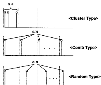
그림 3. OFDM 시스템의 자원할당 방식 Fig. 3. Three type of resource allocation method
