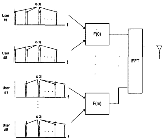
그림 6. 가상 다중안테나 기법을 적용한 하향링크 블록도 Fig. 6. The block diagram of downlink employing subcarrier-based virtual multiple antenna.
