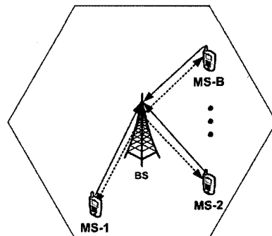
그림 5. 부반송파 기반의 가상 다중안테나 기법을 이용한 SDMA Fig. 5. SDMA using subcarrier-based virtual multiple antenna.
