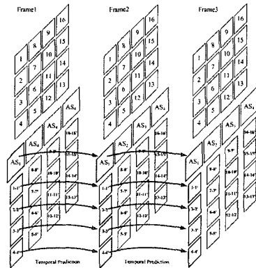
그림 9. 홀로그래프 비디오의 시간적 예측 기술 Fig. 9. Temporal prediction technique of hologram video
