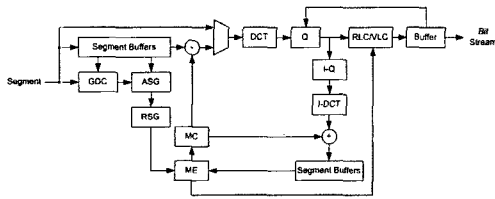
그림 10. 집적영상 기반의 다시점 부호화기 Fig. 10. Multi-view codec based accumulated segment
