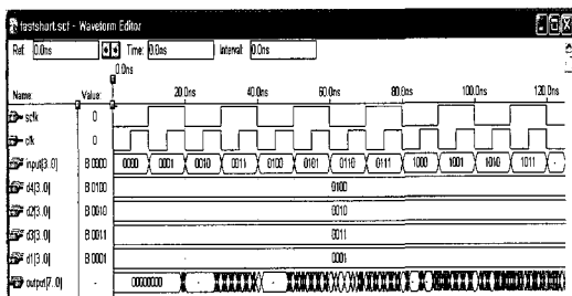
그림 22. h(-n), g(-n) 의 Time Simulation
