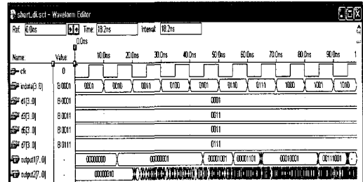
그림 25. h(n), g(n) 의 Time Simulation
