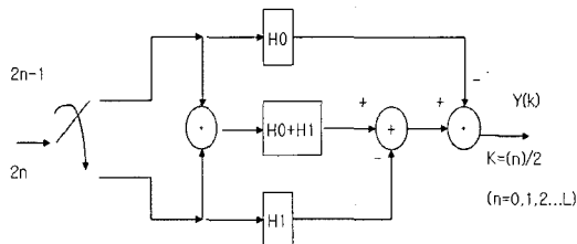
홀수부분의 출력 과정을 생략한 알고리즘
