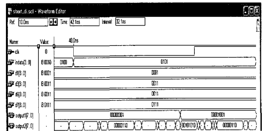
그림 26. h(n), g(n) 의 Time Simulation의 확대모습
