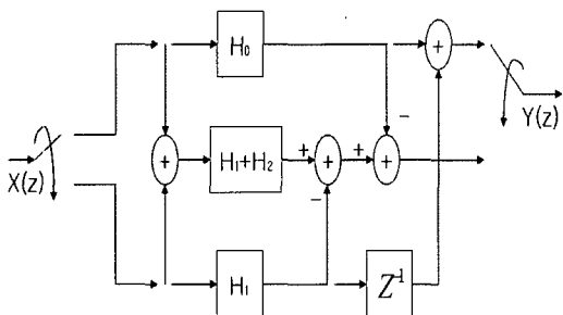
그림 9. short-length running FIR 알고리즘
