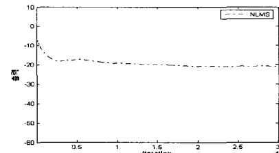
NLMS의 MSE
