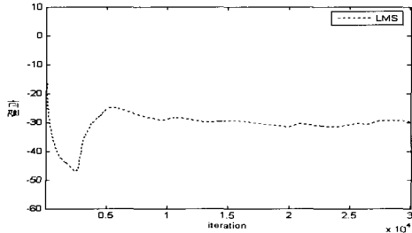
LMS의 MSE
