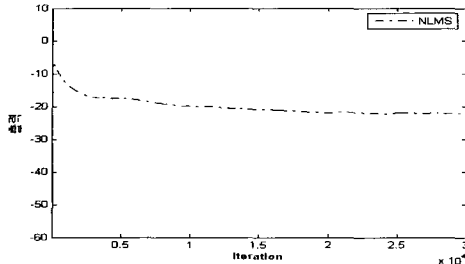
NLMS의 MSE
