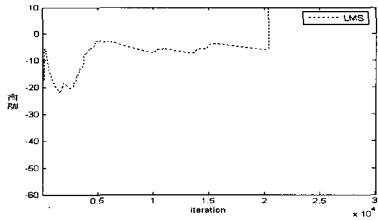
LMS의 MSE
