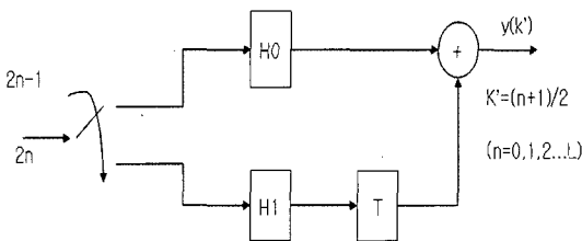
짝수부분의 출력 과정을 생략한 알고리즘
