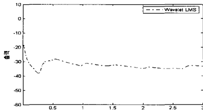
wavelet LMS의 MSE
