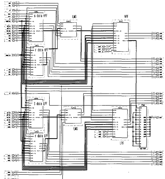
그림 19. Graphic editor로 나타낸 적응 등화기의 구조
