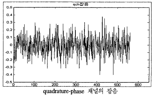
그림 13. 각각의 채널 잡음
