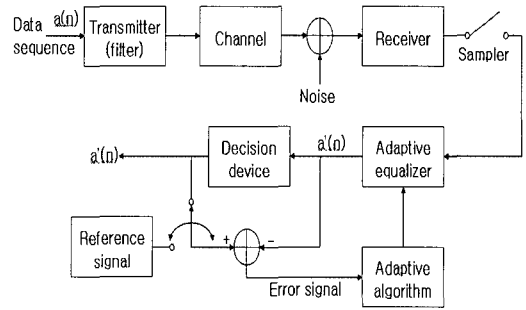
그림 6. 등화기 블록도
