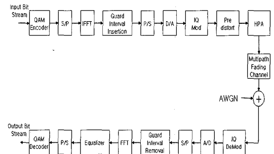
그림 5. OFDM 전송 시스템 구성도
