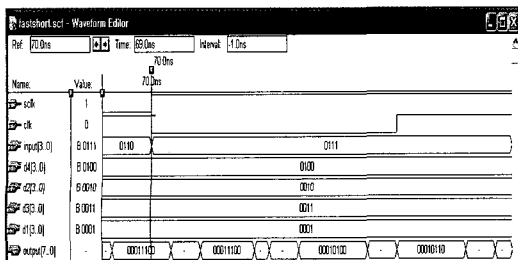
그림 23. h(-n), g(-n) 의 Time Simulation의 확대모습
