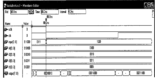
그림 24. h(-n), g(-n) 의 Time Simulation의 확대모습
