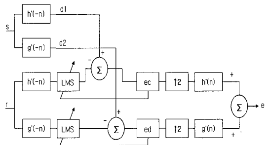
그림 10. 웨이블릿 기반에 제안한 고속화 알고리즘을 적용한 구조
