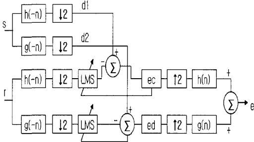
그림 7. 웨이블릿 기반 적응 알고리즘에 대한 구조
