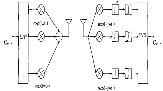
그림 4. OFDM의 기본 구조
