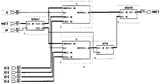
그림 20. 간략화한 h(-n), g(-n) 의 구조
