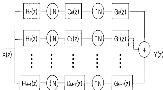
그림 8. 일반적인 M차 멀티레이트 분석·합성 필터뱅크
