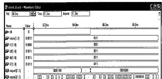
그림 27. h(n), g(n) 의 Time Simulation의 확대모습
