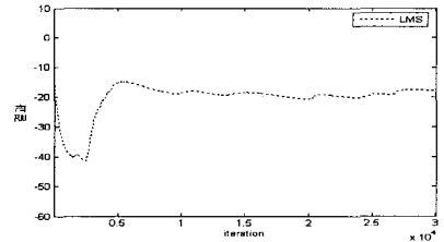
LMS의 MSE
