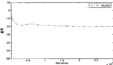
NLMS의 MSE
