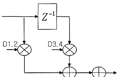
그림 10. short-length running FIR 알고리즘의 필터
