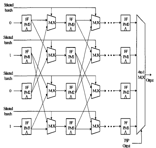
그림 6. PR(121)의 RE 방식에 대한 RTL 블록도
