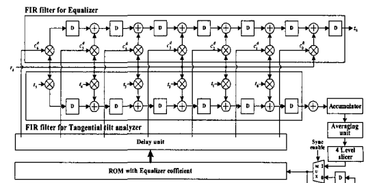
그림 2. 디스크 기울임 각도 분석기를 갖는 등화기 구조
