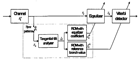
그림 1. 제안한 PRML 검출기의 전체 블록도
