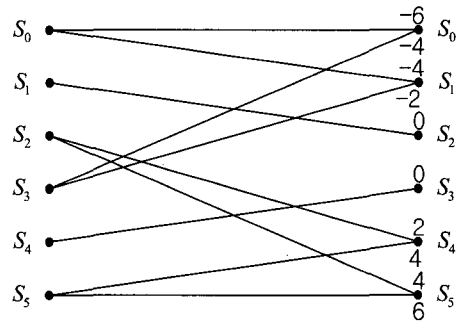
그림 5. PR(1221)의 트렐리스
