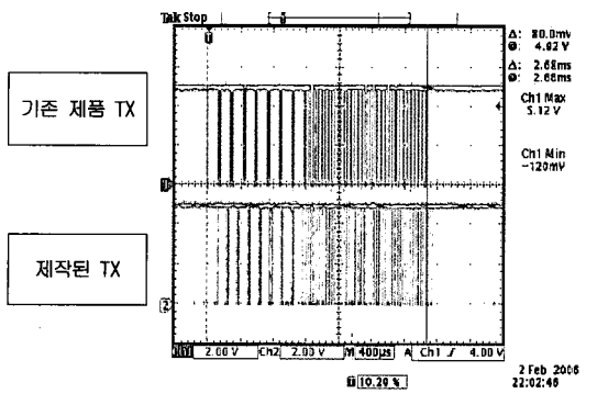
그림 8. 제작된 TX와 기존 제품 TX 비교 파형
