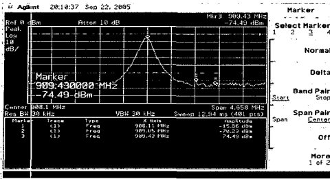
그림 14. ① RF_OUT 출력파형
