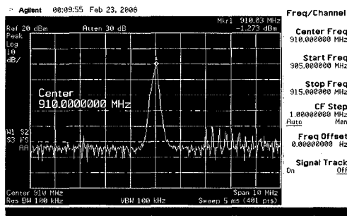
그림 25. TX (U108-1-PIN)출력
