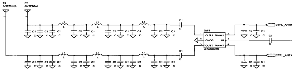
그림 11. RFID 수신부 회로도 (기존 제품)
