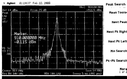
그림 24. TX (U106-8-PIN)출력
