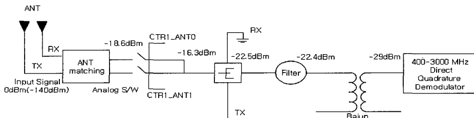
그림 12. RFID 송·수신부 시스템 블록도 (기존 제품)
