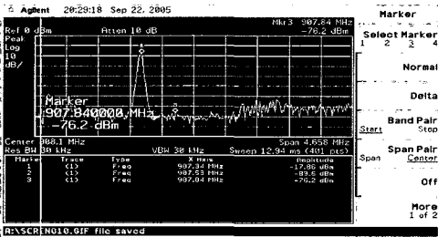
그림 15. ② RF_OUT 출력파형
