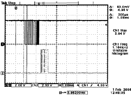
그림 5. RFID 리더기가 Power ON 되고 Read 명령이 있을 때 분석 파형(기존 제품)
