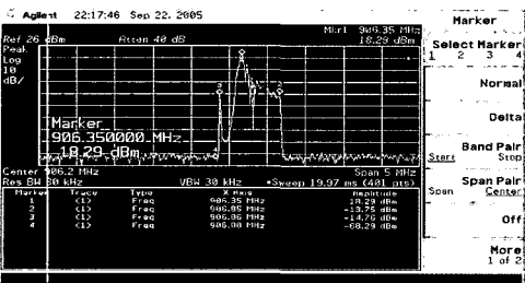
그림 17. ⑥ RF_OUT 출력파형
