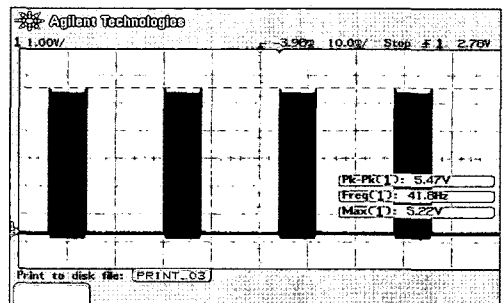
그림 21. RX 데이터 측정(RXD0)
