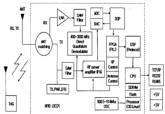
그림 2. 수동형 RFID 리더기 전체 구성도
