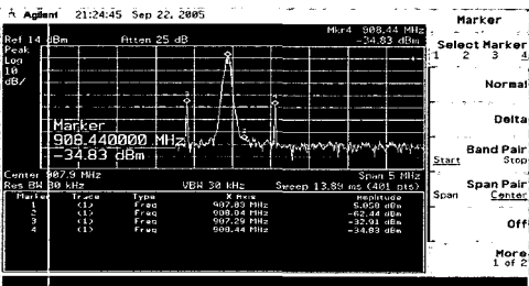
그림 16. ④ RF_OUT 출력파형
