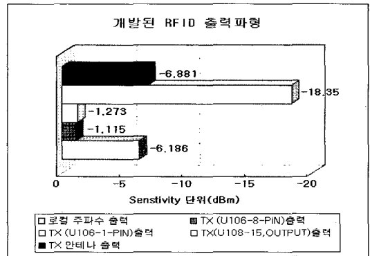
그림 28. 개발된RFID 출력 파형
