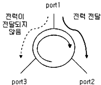
그림 3. 포트에 전력이 들어간 경우
