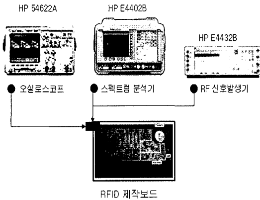
그림 10. 실험 구성도
