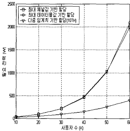
그림 5. 사용자 수에 따른 제안된 알고리즘과 기존 알고리즘들의 평균 CPU 처리 시간
