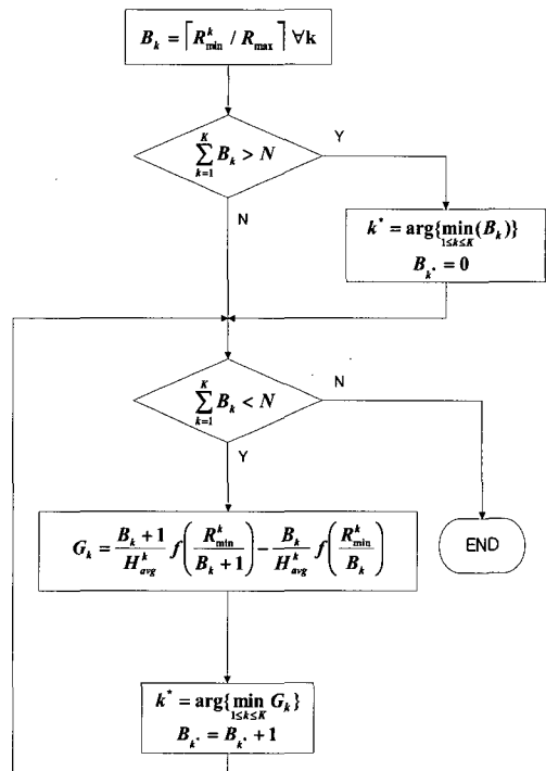
그림 1. 요구 데이터율 기반 대역폭 할당 알고리즘
