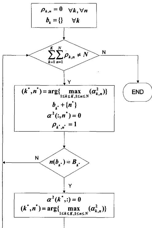
그림 2. 최대 채널값 기반 부반송파 할당 알고리즘
