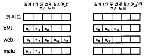
(b) 분할 인덱스
