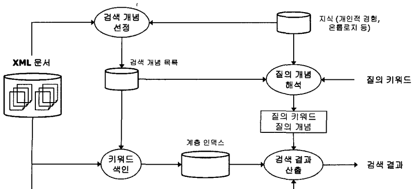
그림 1 의미 기반 키워드 검색 개요
