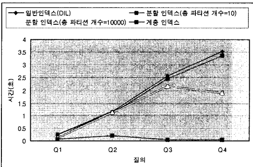
그림 8 DBLP XML 문서에 대한 검색 소요 시간
