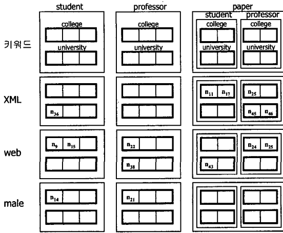
(a) 의미 기반 계층 인덱스
