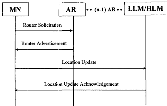
(그림 7) Q.MMF 경우1의 위치등록절차
