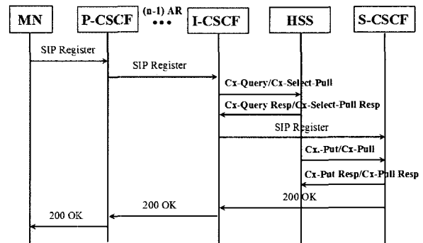
(그림 10) IMS 위치등록절차
