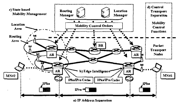
(그림 3) IP2 이동성 관리 구조
