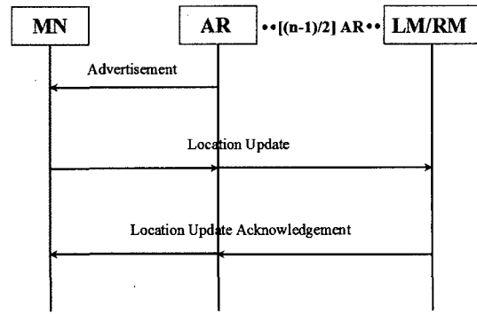
(그림 5) IP2 경우2의 위치등록절차
