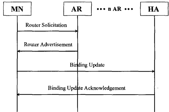
(그림 2) MIPv6 위치등록절차
