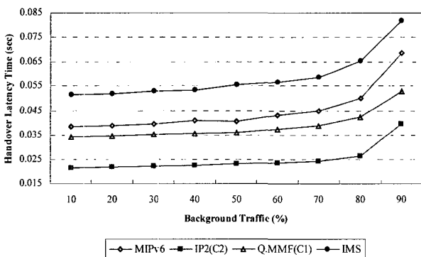
(그림 17) 백그라운드 트래픽의 증가에 따른 핸드오버지연 시간의 변화
