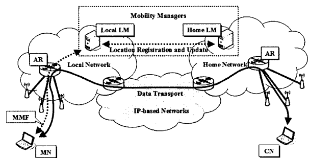
(그림 6) Q.MMF 이동성 관리 구조
