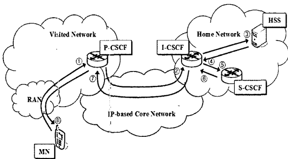
(그림 9) IMS 이동성 관리 구조
