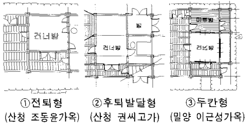
그림 13. 안채 건너방 유형
