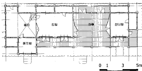
그림 2. 정지부분-두칸형 (밀양 손용상가옥 안채평면도)
