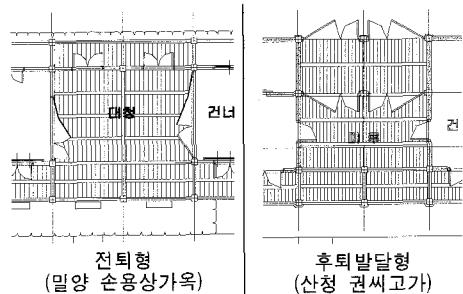
그림 7. 안채 마루부분 평면유형
