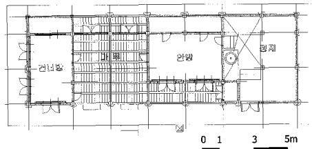
그림 4. ‘두칸+퇴칸’형 밀양 손영배가옥 안채평면도
