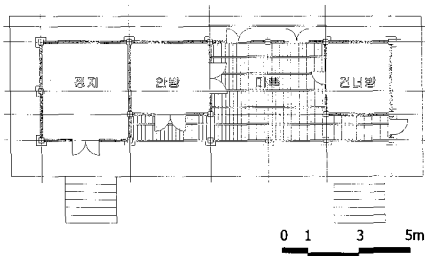
그림 1. 전퇴형(고성 최영덕가옥 평면도)
