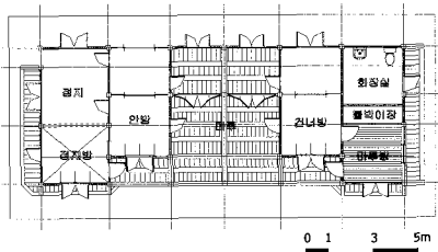
그림 6. 정지 건너방부분 두칸형 (창녕 성씨고가 안채 평면도)
