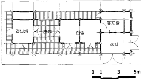
그림 12. 함안 이씨고가 안채평면도
