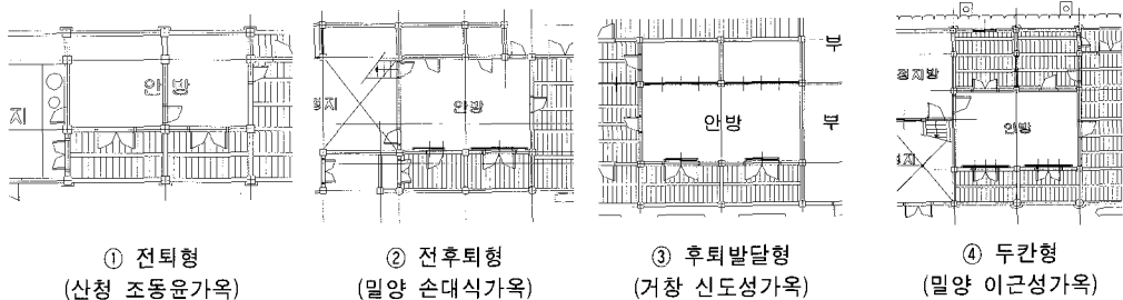
그림 10. 안방 평면유형
