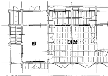
그림 8. 밀양 손병구 가옥 안채 마루부분 평면도
