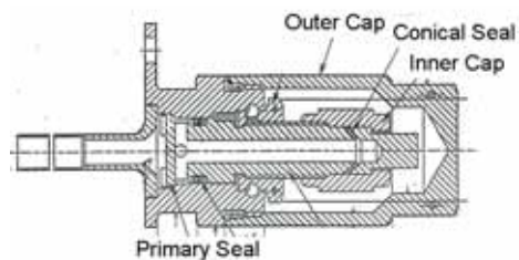
그림 2. Fill/Drain Valve using Disk Type Primary Seal
