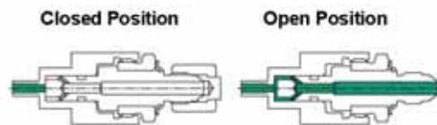
그림 1. Operating Configuration of Fill/Drain Valve
