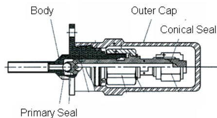
그림 3. Fill/Drain Valve using Ball Type Primary Seal
