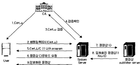
(그림 3) 사용자 인증 프로토콜
