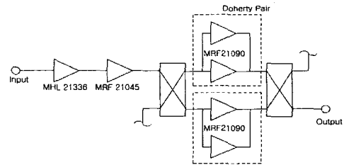
그림 5. GCHD 전력증폭기의 블록도 Fig. 5. The block diagram of GCHD PA.
