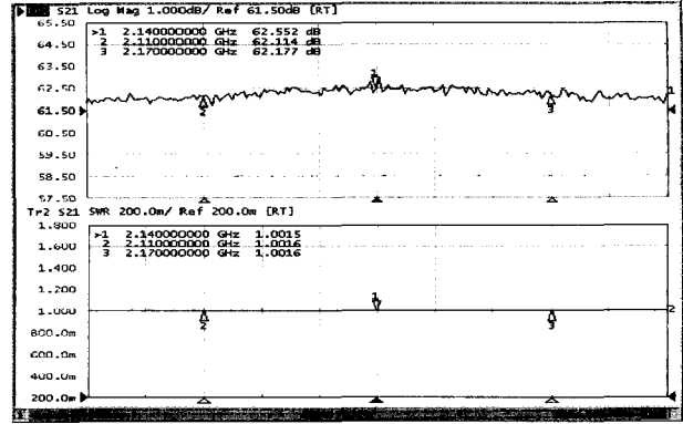
그림 14. GCHD 전력증폭기의 이득특성 Fig. 14. The gain characteristic of GCHD PA.
