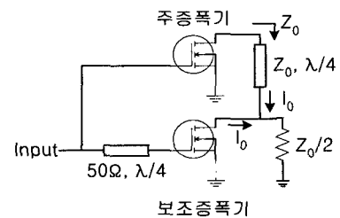
(b) 최대 입력전력레벨 동작모드
