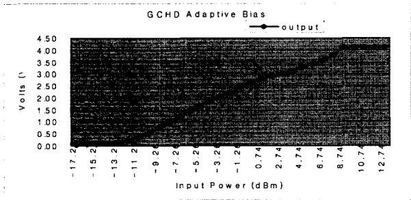
그림 13. Gate 바이어스 조절회로의 출력특성 Fig. 13. The output characteristic of Gate bias control.
