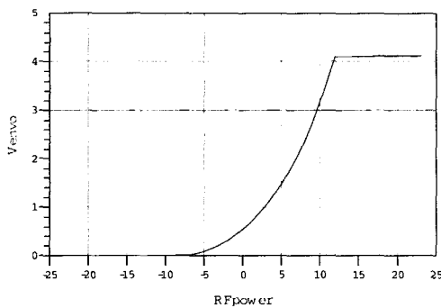
그림 9. Gate 바이어스 제어부의 출력특성 Fig. 9. The output characteristic of Gate bias control.
