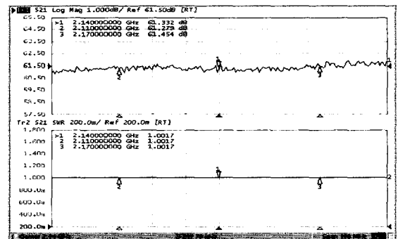
그림 11. Doherty 전력증폭기의 이득특성 Fig. 11. The gain characteristic of general Doherty PA.
