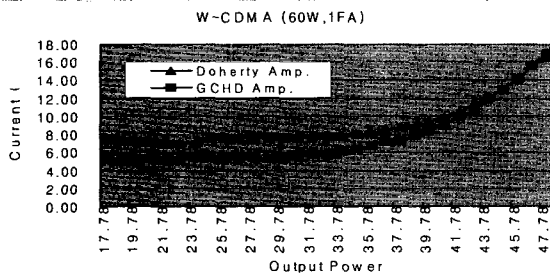
그림 17. GCHD 전력증폭기의 소비전류비교 Fig. 17. The comparison of current consumption.
