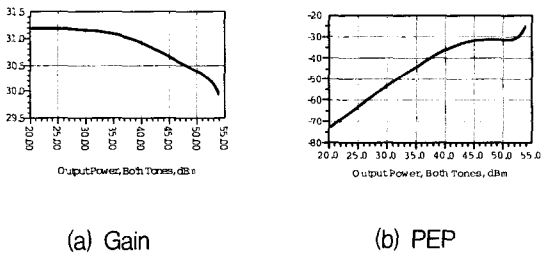
그림 8. Doherty 전력증폭기의 출력특성 Fig. 8. The output characteristics of Doherty PA.
