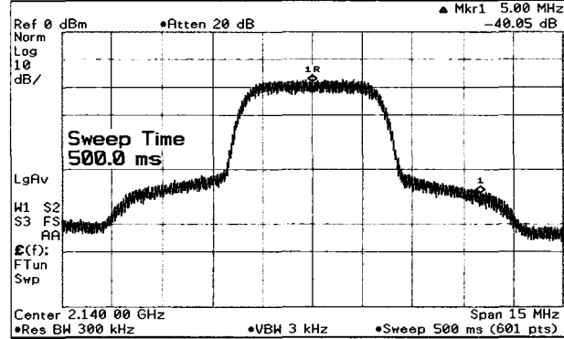
그림 15. GCHD 전력증폭기의 ACLR 출력특성 Fig. 15. The ACLR characteristic of GCHD PA.
