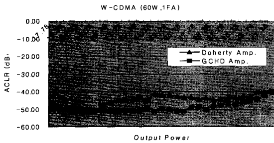
그림 16. GCHD 전력증폭기의 ACLR 출력특성비교 Fig. 16. The comparison of ACLR characteristics.
