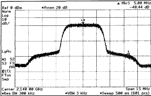
그림 12. Doherty 전력증폭기의 ACLR 출력특성 Fig. 12. The ACLR characteristic of general Doherty PA.
