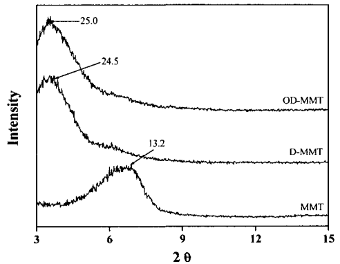
Fig. 2 XRD of MMT, D-MMT, and OD-MMT.
