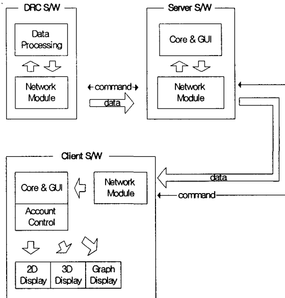
< 그림 2 > 전체 소프트웨어 구조
