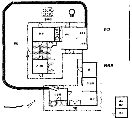
그림 15. 이경식씨 집 평면
