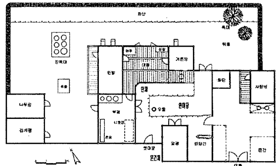
그림 6. 김병선씨 집 평면
