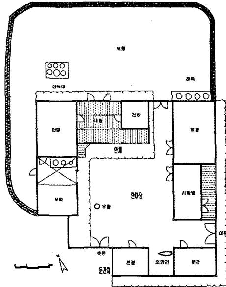
그림 26. 이병출씨 집 평면
