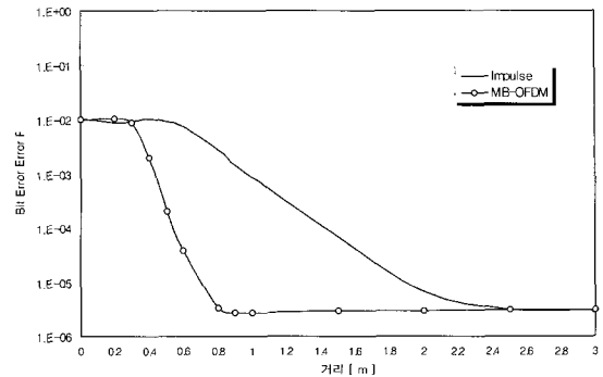
그림9. 위성직접수신DMB의 UWB 간섭원의 거리에 따른 BER 특성 (no UWB: 10^{-7} 이하, SDMB 수신레벨:-95dBm)
