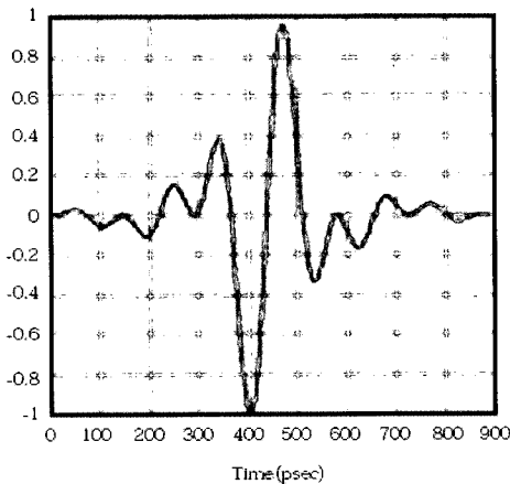
그림1. 시간축에서 본 UWB 펄스신호
