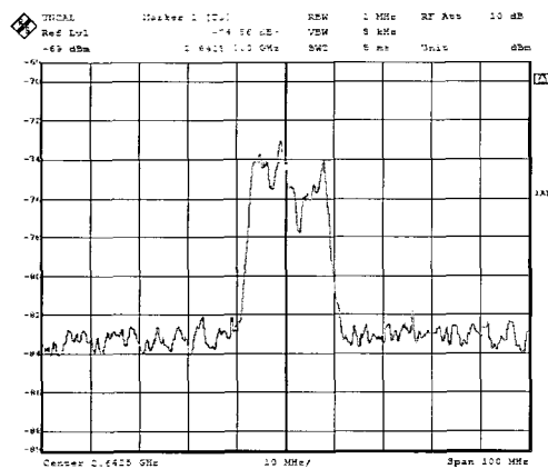
그림8. SDMB Gap-Filler 수신신호
