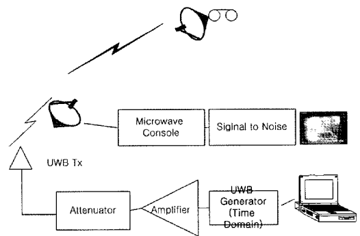
그림5. 방송중계망 전파간섭측정 구성도
