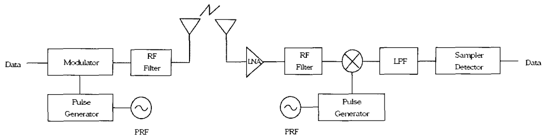
그림 2. UWB 송수신기 구조
