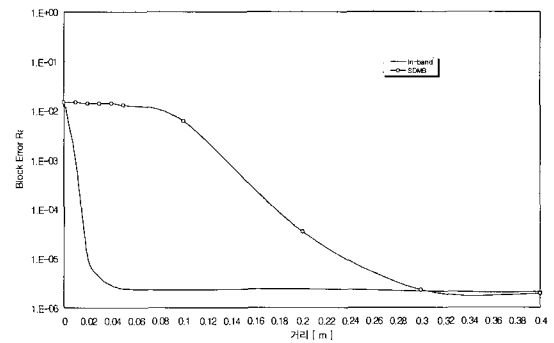
그림10. Gap-Filler수신 DMB의 UWB 간섭원의 거리에 따른 BER 특성 (no UWB: 10^{-7} 이하, Gap-Filler수신레벨:-70dBm)
