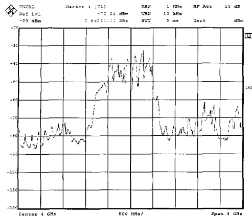
그림 6. OFDM 방식 UWB 출력파형
