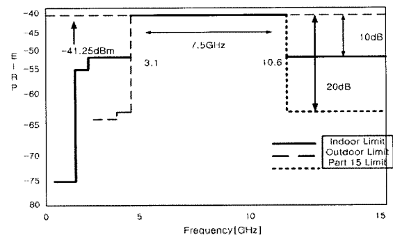
그림3. UWB 신호에 대한 규격
