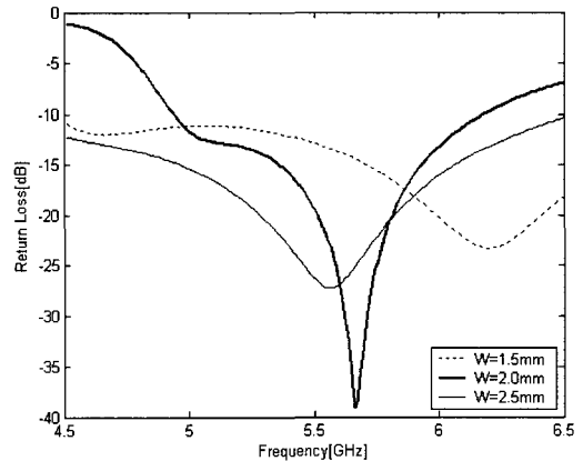
그림 4. 미앤더 선로의 폭 W 의 변화에 따른 반사 계수 Fig 4. Influence of the width of W on the return loss of the proposed antenna
