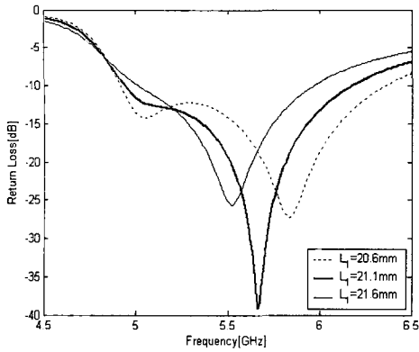
그림 5. 미앤더 선로의 길이 L_1 의 변화에 따른 반사 계수 Fig 5. Influence of the width of L_1 on the return loss of the proposed antenna
