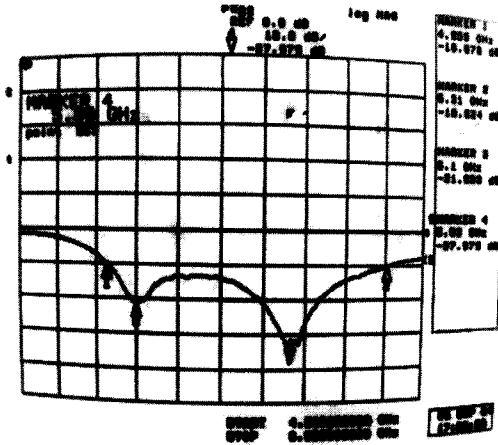
그림 11. 측정된 반사계수 Fig 11. Measured return loss vs. frequency for the proposed antenna
