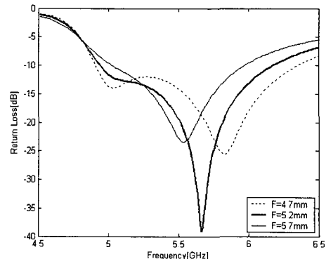
그림 8. 동축 급전의 위치 F 의 변화에 따른 반사 계수 Fig 8. Influence of the width of F on the return loss of the proposed antenna
