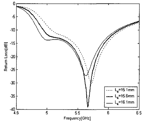
그림 7. 미앤더 선로의 길이 L_4 의 변화에 따른 반사 계수 Fig 7. Influence of the width of L_4 on the return loss of the proposed antenna
