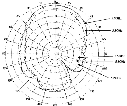
(b) H-평면
