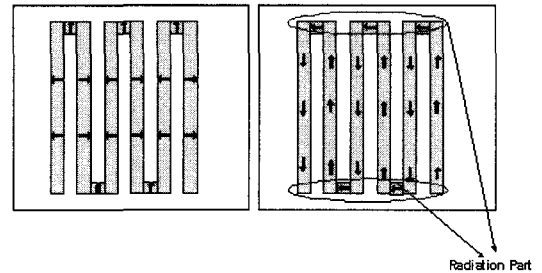
그림 1. 미앤더 선로의 전기분포와 자기분포 Fig 1. Electric field and Magnetic field of Meander railroad
