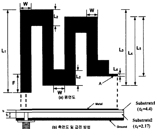
그림 3. 제안된 안테나의 구조 Fig 3. Configuration of the proposed antenna (a) top vies (b) side view
