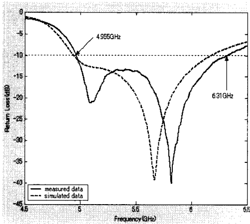
그림 12. 실제 측정된 반사계수와 시뮬레이션된 반사계수 Fig 12. Measured return loss vs. Simulated return loss
