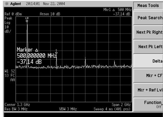
그림 11. FP ROF 링크의 RF 캐리어의 고조파 성분 Fig. 11. High-order harmonics of RF carrier of FP ROF link.
