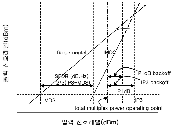
그림 1. SFDR 특성 Fig. 1. Characteristics SFDR.
