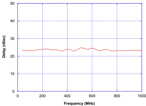
그림 13. 측정된 FP ROF 링크의 지연시간 Fig. 13. Measured delay time of FP ROF link.
