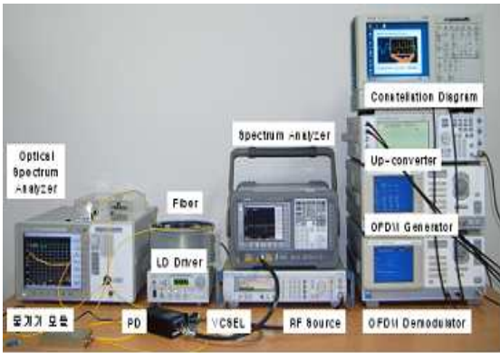
그림 10. ROF 링크 특성 측정 실험 구도 Fig. 10. The configuration to test ROF link characteristics.
