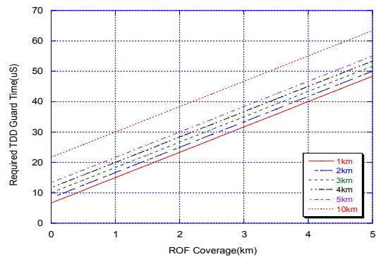
그림 9. 중계 거리에 따른 TDD 가드 시간 Fig. 9. Calculated TDD guard time in terms of link length
