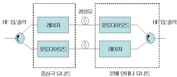
그림 4. 전형적인 ROF 시스템 구조. Fig. 4. A typical ROF system configuration.
