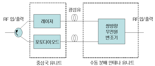
그림 5. 제안한 PIP 구조. Fig. 5. The proposed PIP configuration.
