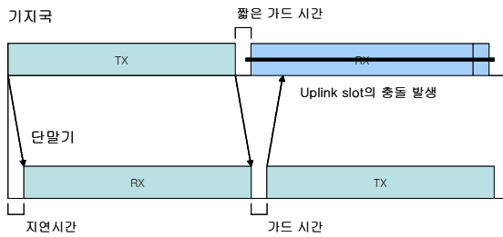
그림 6. TDD 가드 시간이 짧은 경우 프레임의 충돌 Fig. 6. Congested frame in case of short TDD guard time.
