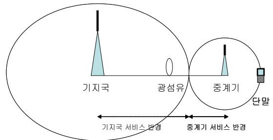
그림 8. ROF 중계기 지연 시간 계산을 위한 구도. Fig. 8. Configuration for calculating delay time of ROF link.
