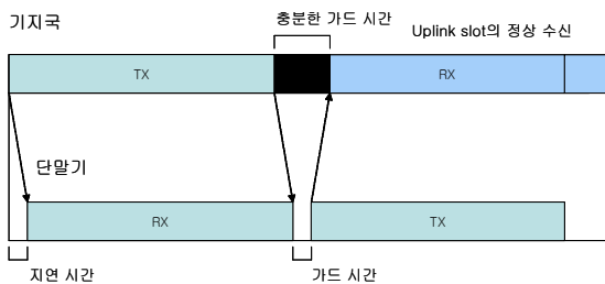
그림 7. TDD의 가드 시간이 충분한 경우상향 및 하향 프레임 Fig. 7 Up-link and down-link frame in case of enough TDD guard time.
