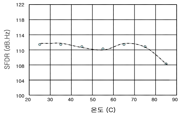
그림 2. FP ROF의 온도에 따른 SFDR 특성 Fig. 2. SFDR characteristics of a FP ROF link vs temperature.
