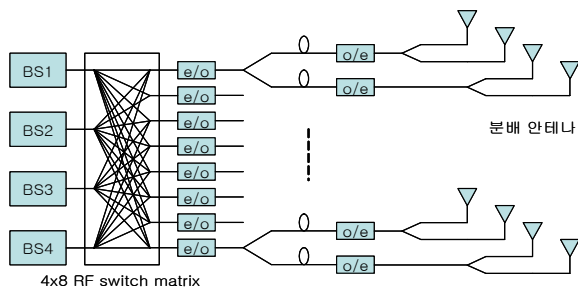
그림 3. 안테나 분배시스템(4개의 기지국, 32개의 분배 안테나)
