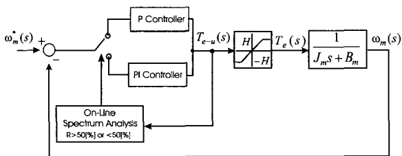
그림 5 제안된 anti-windup 전체 블럭도 Fig. 5 Block diagram of proposed anti-windup scheme
