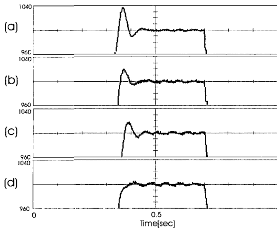
그림 16 스텝 속도 지령에 대한 확대된 비교 응답 파형: (a) 조건부 적분 기법, (b) Back-calculation 기법, (c) 하이브리드 기법, (d) 제안된 기법 Fig. 16 Comparison of speed performance for step speed command:(a) Conditional Integration Scheme, (b) Back-calculation Scheme, (c) Hybrid Scheme, (d) Proposed Scheme
