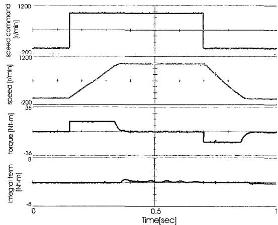
그림 14 1000 r/min 스텝 속도 지령에 대한 제안된 기법의 응답 파형
