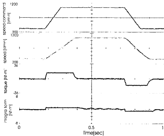
그림 13 1000 r/min 램프 속도 지령에 대한 제안된 기법의 응답 파형
