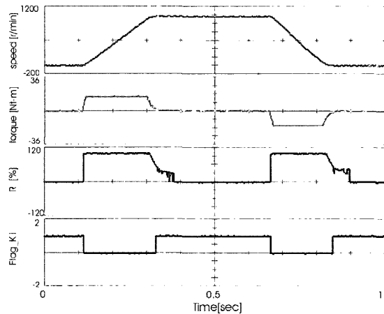
그림 15 제안된 기법의 Spectral Energy Ratio 및 제어기 절환 플래그
