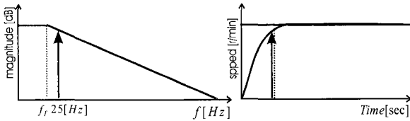
그림 6 시간 영역에서 본 f_T 와 주파수 영역에서 본 f_T 선택의 차이 비교 Fig. 6 Influence for selection of break frequency in frequency and time domain
