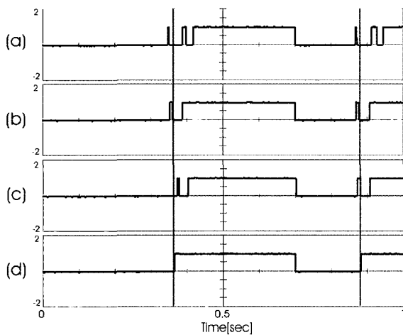
그림 17 정착시간 비교 결과:(a) 조건부 적분 기법, (b) Back-calculation 기법, (c) 하이브리드 기법, (d) 제안된 기법 Fig. 17 Comparison of settling time:(a) Conditional Integration Scheme, (b) Back-calculation Scheme, (c) Hybrid Scheme, (d) Proposed Scheme
