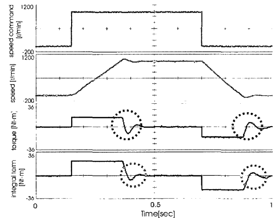
그림 8 1000 r/min 스텝 속도 지령에 대한 조건부 적분 기법의 응답 파형 Fig. 8 Responses of conditional integration scheme for 1000 r/min step speed command
