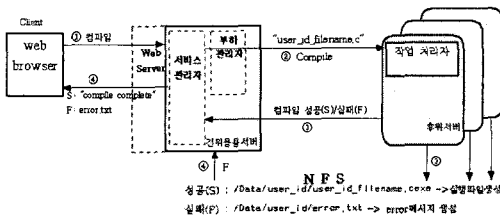
그림 10. 저장된 과제 컴파일 수행 절차
