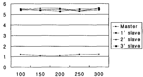
그림 4. Request 수 증가에 따른 응답속도
