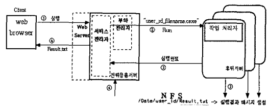
그림 9. 컴파일된 과제의 실행 절차
