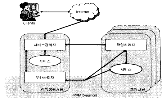
그림 2. 구현된 시스템 구성도
