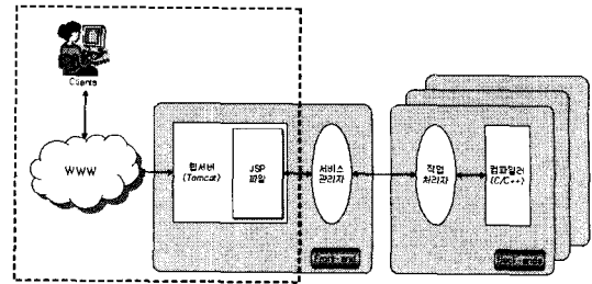
그림 8. 응용서비스 시스템 구성
