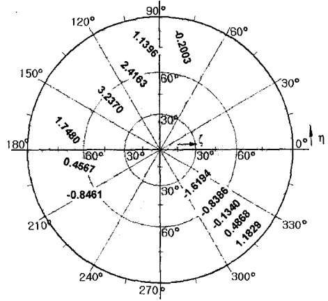
그림 1. [\bar{1}11] 방향으로 전기장을 가할 경우 나타나는 굴절률 변화의 입체투영도( \times 10^{-11} V^{-1} ).
