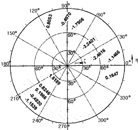
그림 3. [111] 방향으로 전기장을 가할 경우 나타나는 굴절률 변화의 입체투영도( \times 10^{-11} V^{-1} ).
