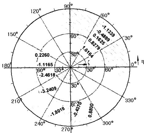
그림 4. [\bar{1}\bar{1}\bar{1}] 방향으로 전기장을 가할 경우 나타나는 굴절률 변화의 입체투영도( \times 10^{-11} V^{-1} ).
