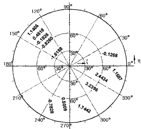
그림 2. [1\bar{1}\bar{1}] 방향으로 전기장을 가할 경우 나타나는 굴절률 변화의 입체투영도( \times 10^{-11} V^{-1} ).
