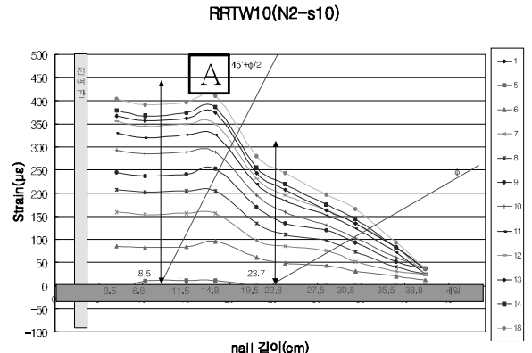
그림 6 벽체 회전 인발 시험(200 kgf)
