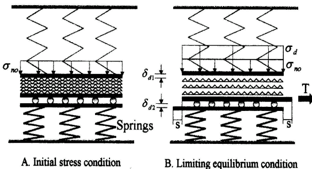
그림 1 구속된 딜리턴시의 모델.
