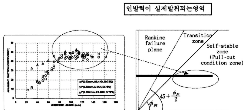
그림 3 변이 영역의 존재. K.T.Chang(1996).
