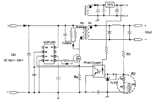
그림 2 온도가 상승할 때 출력전압이 감소하는 DC-DC Converter Fig. 2 Circuit diagram of DC-DC Converter
