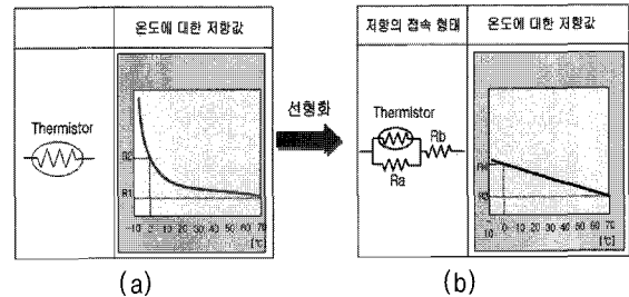
그림 1 NTC 써미스터의 선형화 Fig. 1 Linearization Of NTC Thermistor
