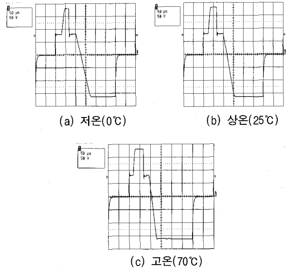
그림 9 저온, 상온, 고온에서의 Reset 전압 파형 Fig. 9 Experiment Result Of Reset Circuit
