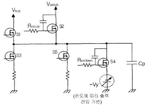
그림 5 온도가 상승할 때 -V_y 전압이 가변되는 Reset 회로 Fig. 5 Circuit diagram of Reset Circuit ( -V_y Voltage Vaies when Temperature rises)
