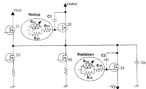
그림 6 온도가 상승할 때 기울기가 증가하는 Reset 회로 Fig. 6 Circuit diagram of Reset Circuit(The Slope rate Of Ramp Voltage increases when Temperature rises)
