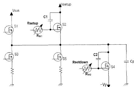
그림 7 온도가 상승할 때 기울기가 감소하는 Reset 회로 Fig. 7 Circuit diagram of Reset Circuit(The Slope rate Of Ramp Voltage decreases when Temperature rises)
