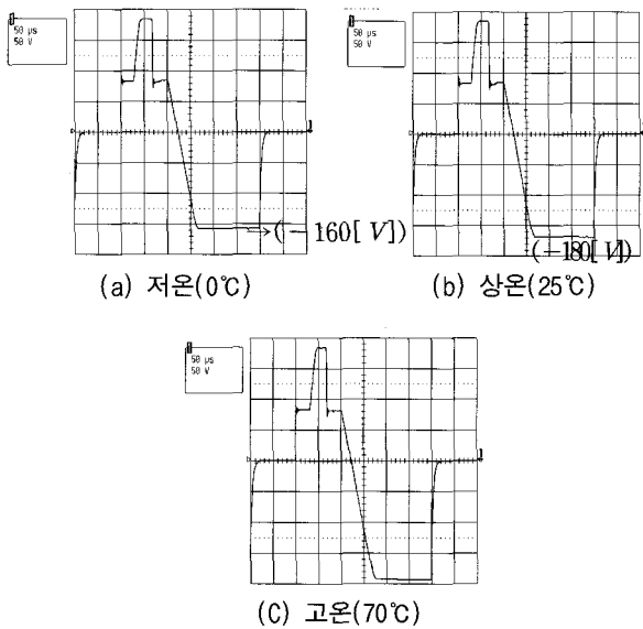
그림 8 저온, 상온, 고온에서의 Reset 전압 파형 Fig. 8 Experiment Result Of Reset Circuit
