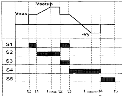
그림 3 Reset 파형의 스위치 시간별 동작모드 Fig. 3 Switch Signal Of Reset Waveforms
