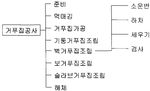
그림 2. 거푸집 공사 공종분할의 예
