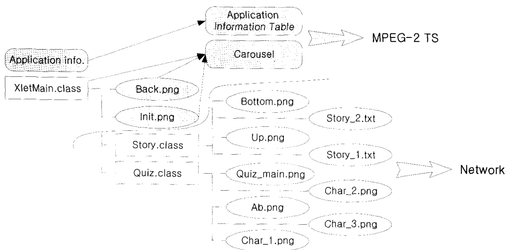
(그림 4) 통방융합 데이터방송 서비스를 위한 콘텐츠 구조의 예
