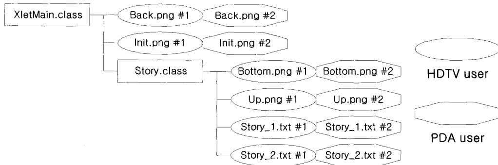
(그림 5) 데이터방송의 타겟팅 서비스를 위한 콘텐츠 구조의 예
