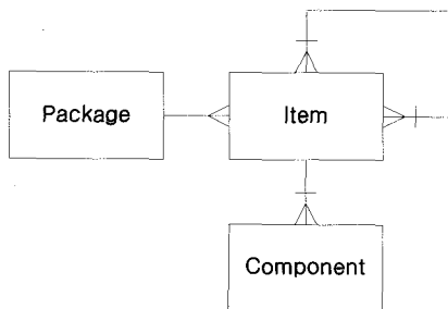
(그림 1) 패키지 모델의 논리 구조
