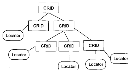
(그림 2) CRID, Locator 관계의 예
