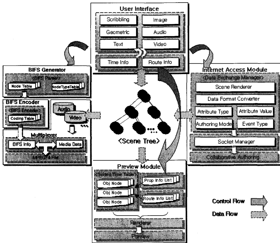
(그림 1) MPEG-4 저작 시스템 구조
