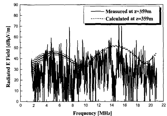
그림 17. CD 중간지점 ( z=359m, y=1.2m ) 에서 방사전계 측정치 및 계산치 Fig. 17. Measured and calculated value of radiated electric field at center point between C and D ( z=359m, y=1.2m ).
