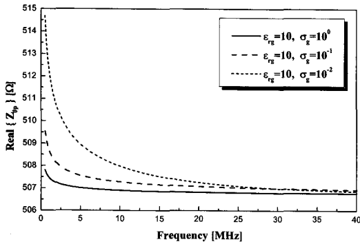
그림 4. \epsilon_{rg}=10 일 때 지면 도전율의 변화에 따른 특성 임피던스
