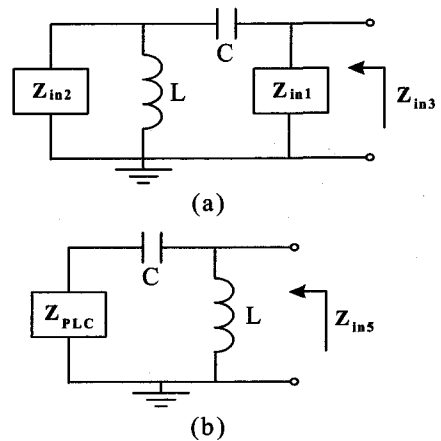
그림 2. (a) Z_{in3} 계산을 위한 등가회로 (b) Z_{in5} 계산을 위한 등가회로 Fig. 2. (a) Equivalent circuit for Z_{in3} calculation, (b) Equivalent circuit for Z_{in5} calculation.
