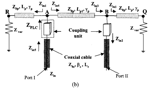
그림 1. (a) 전력선 통신 시스템의 구성도 (b) 2포트 등가모델 Fig. 1. (a) A schematic configuration of PLC system. (b) 2port equivalent model.
