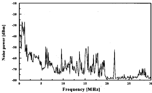
그림 7. 측정된 전도성 잡음 Fig. 7. Measured conductive noise.
