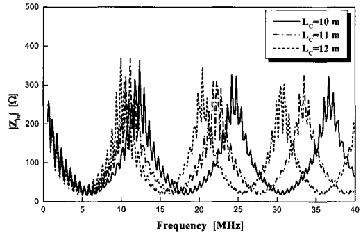
그림 6. \epsilon_{rg}=10, \sigma_g=10^{-1} [S/m] 일 때 L_c 의 변화에 따른 Z_{in}
