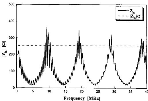
그림 5. \epsilon_{rg}=10, \sigma_g=10^{-1} [S/m] 일 때 Z_{in}
