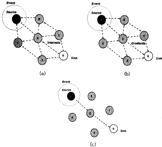
그림 1. Directed Diffusion 알고리즘 동작 과정
