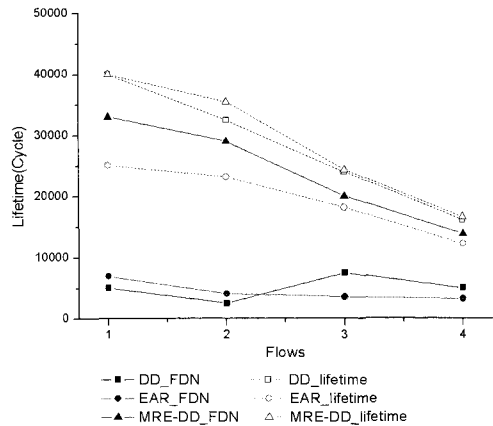
그림 5. 다중 수집노드 네트워크에서 FDN과 lifetime 비교
