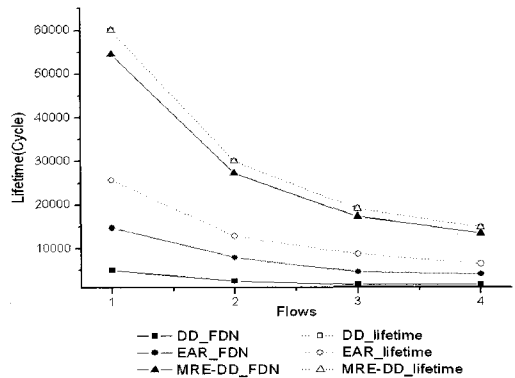
그림 10. FDN과 lifetime 비교
