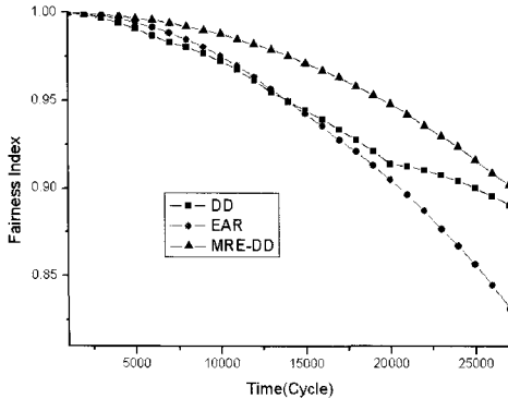
그림 8. 단일 수집노드 네트워크에서 fairness index 비교
