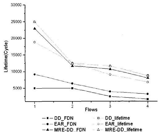
그림 7. 단일 수집노드 네트워크에서 FDN과 lifetime 비교
