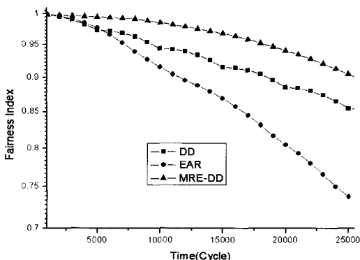
그림 6. 다중 수집노드 네트워크에서 fairness index 비교
