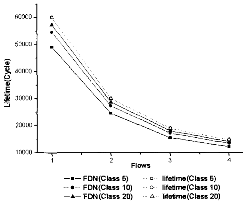
그림 12. MRE-DD 알고리즘 에너지 등급에 따른 FDN과 lifetime 비교
