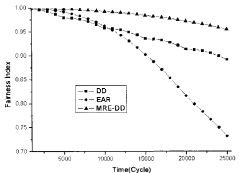
그림 11. Fairness index 비교
