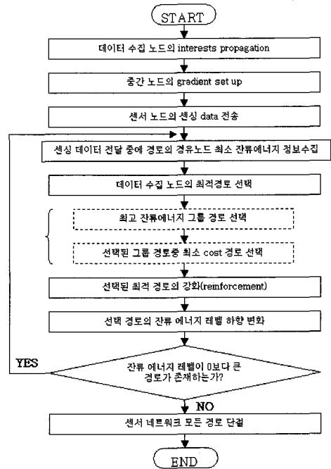
그림 3. MRE-DD 라우팅 알고리즘 절차
