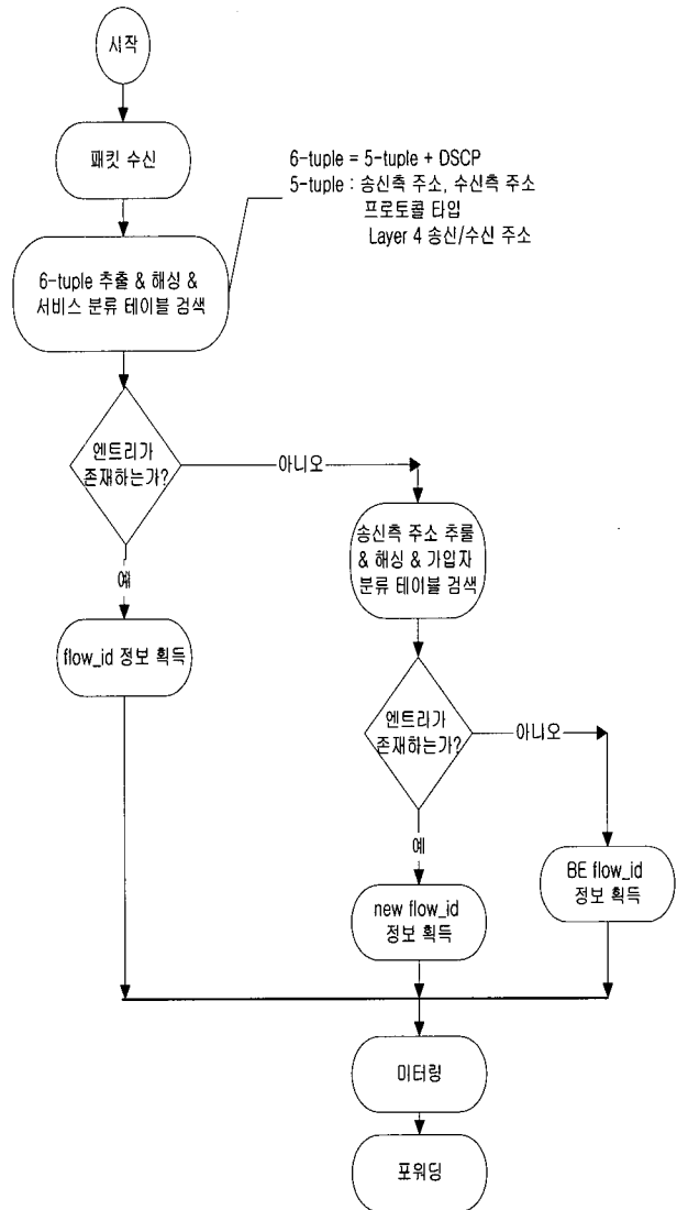
(그림 4) 패킷 분류 절차도
