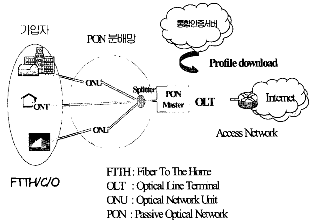
(그림 1) PON 액세스 망의 구조
