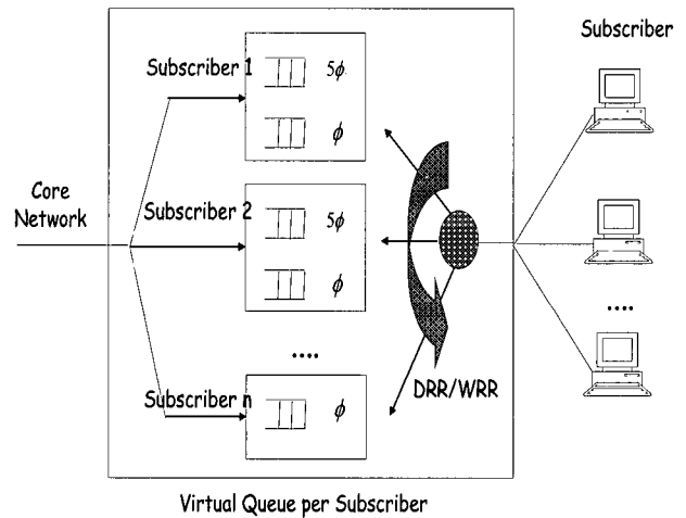
(그림 6) 가입자 단위의 큐잉 및 스케줄링의 예
