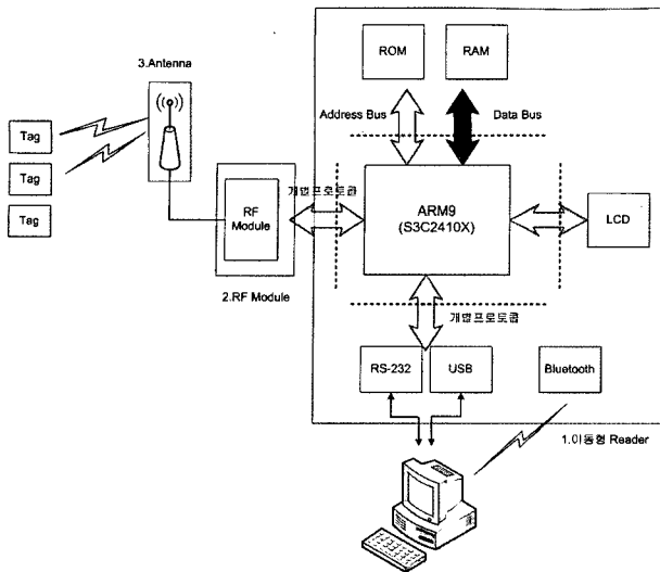
그림 2 이동형 uID Reader Platform 블록도
