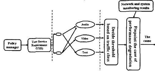
그림 2. QoS 만족도/ 문제점 파악을 위한 과정.
