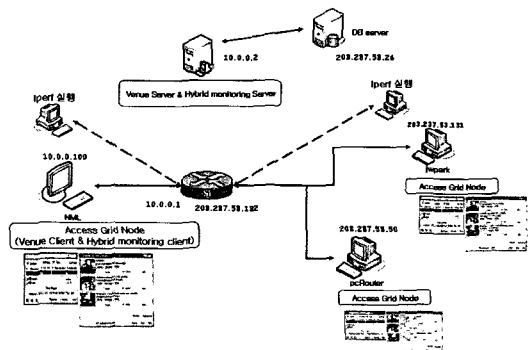
그림 7. 실험 구성도.
