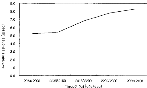
(그림 4) 일반적인 NFS 오퍼레이션 결과 (specSFS97)
