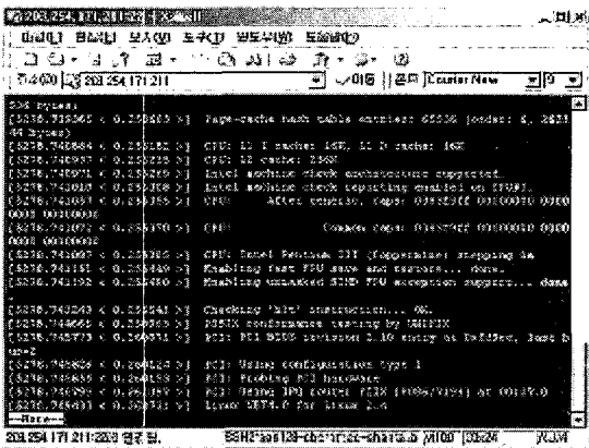
(그림 3) InstrumentedPrintk를 이용한 커널 지연시간 측정
