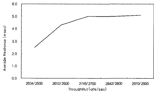
(그림 5) Zero Copy NFS 오퍼레이션 결과 (specSFS97)
