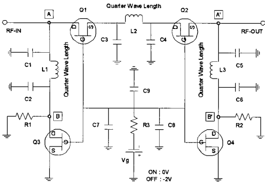
그림 3. 흡수형 MMIC 스위치의 구조 Fig. 3. Configuration of absorptive type MMIC switch.
