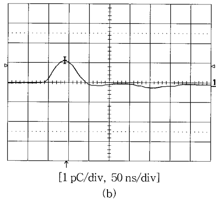
그림 5. 검출된 부분방전 파형 ; (a) AC 660 V peak 인가시, (b) AC 1,040 V peak 인가시.
