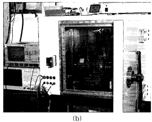
그림 1. 제작한 부분방전 측정시스템 ; (a) 구성도, (b) 사진.
