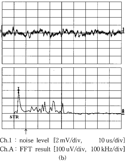
그림 3. PD 측정시스템의 잡음 레벨 평가 ; (a) 개구부 열림, (b) 개구부 닫힘. Fig. 3. Estimation of noise level of the PD measurement system ; (a) door opened, (b) door closed.
