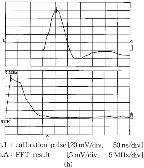
그림 4. 교정 펄스와 주파수 분석 ; (a) 1 pC, (b) 10 pC.
