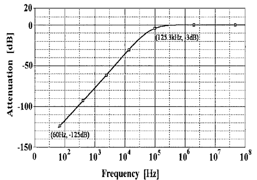
그림 2. 결합 회로망의 주파수 응답특성. Fig. 2. Frequency response characteristic of the coupling network.
