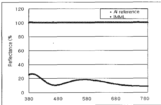
그림 3. 무기금속 다층박막의 반사율. Fig. 3. Reflectance of inorganic multi-layer.
