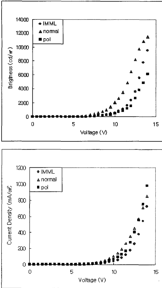
그림 5. 무기금속 다층박막을 적용한 적색 유기발광소자의 I-V-L 특성.
