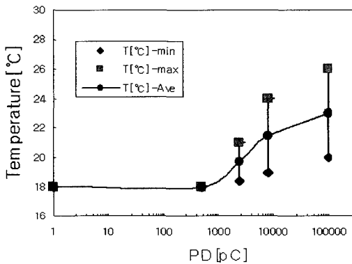
그림 12. BCT에서 PD 와 표면온도 상승특성. Fig. 12. Property of PD and surface temperature increment of BCT.
