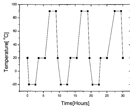
그림 2. 냉열반복 시험.
