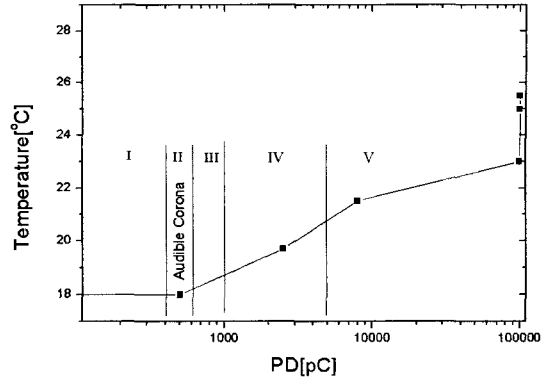
그림 13. 절연열화 기준 특성 곡선. Fig. 13. Example characteristics curve of insulation degradation.
