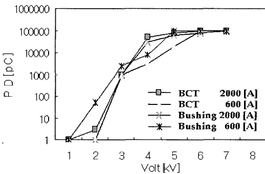
그림 10. 인가전압에 따른 부분방전 특성. Fig. 10. Property of partial discharge dependent on applying voltage.
