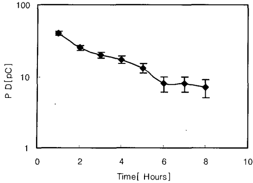
그림 9. 부분방전과 후경화시간 특성. Fig. 9. Property of PD and curing time.
