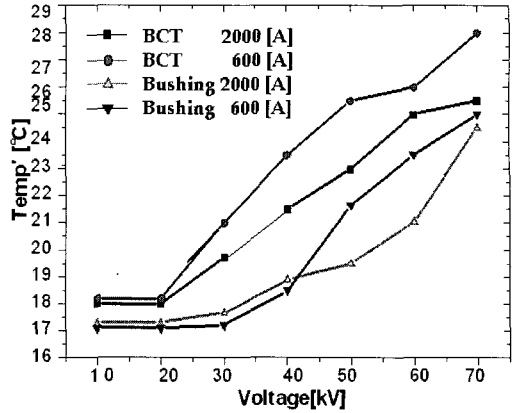
그림 11. 전압인가에 따른 표면온도 상승 특성. Fig. 11. Property of surface temperature increment dependent on applying voltage.
