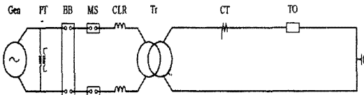
그림 3. 단시간 과전류 강도실험 회로도. Fig. 3. Test Circuit of short time over-current strength.
